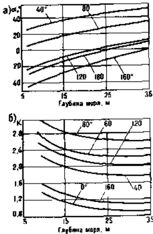
Рисунок 1 - Изменение угла \alpha отклонения направления поверхностных течений (а) и ветрового коэффициента K (б) в зависимости от направления ветра относительно берега и глубины моря (мелководная зона)
